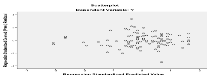
Gambar 2. Uji Heteroskedastisitas
